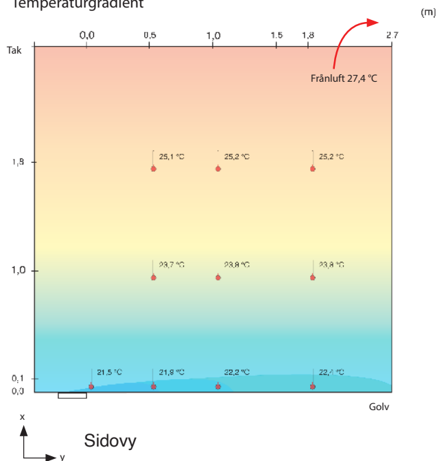
Temperaturgradient
